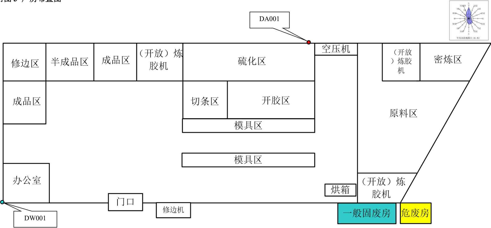
附图 3 厂房布置图
