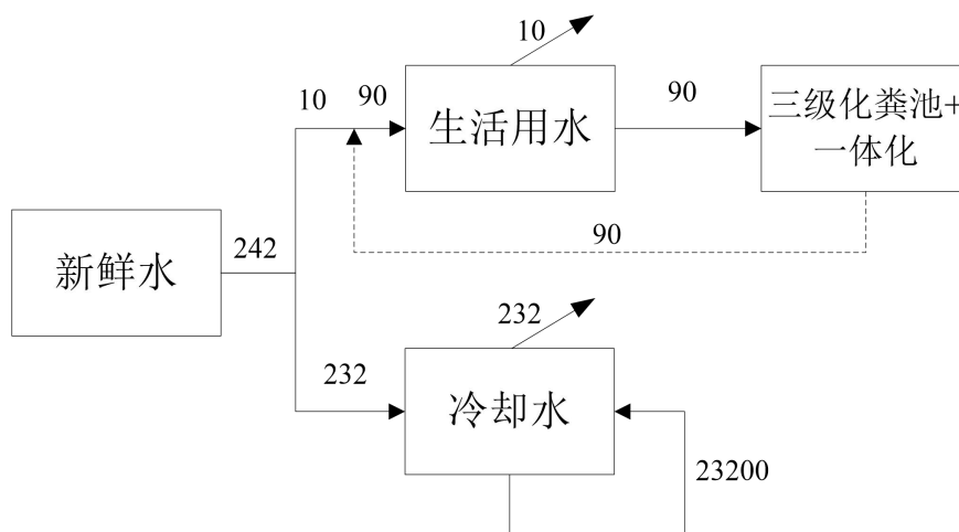
图2-1 项目水平衡图 (m³/a)
