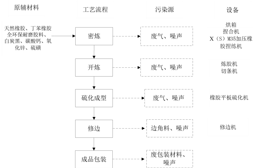
图 2-2 橡胶垫圈生产工艺流程图
