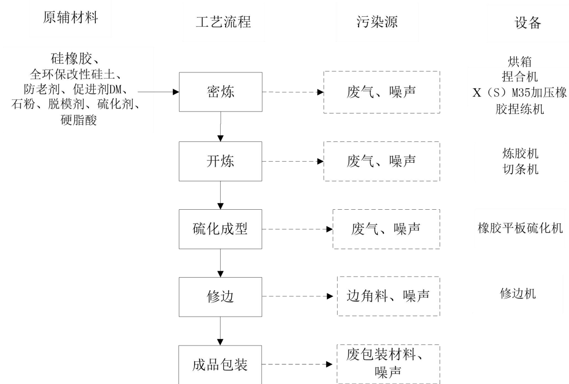
图 2-3 硅胶垫圈生产工艺流程图 1
